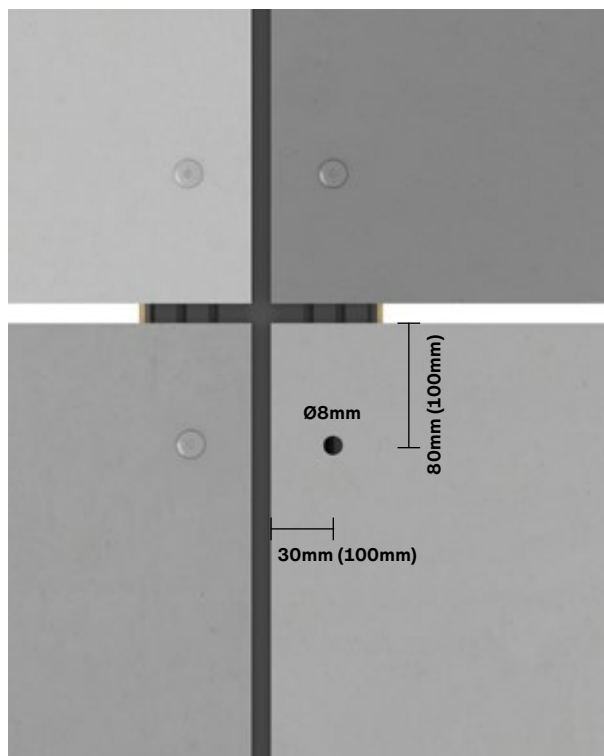
Vertikālās balsta konstrukcijas piemērs
