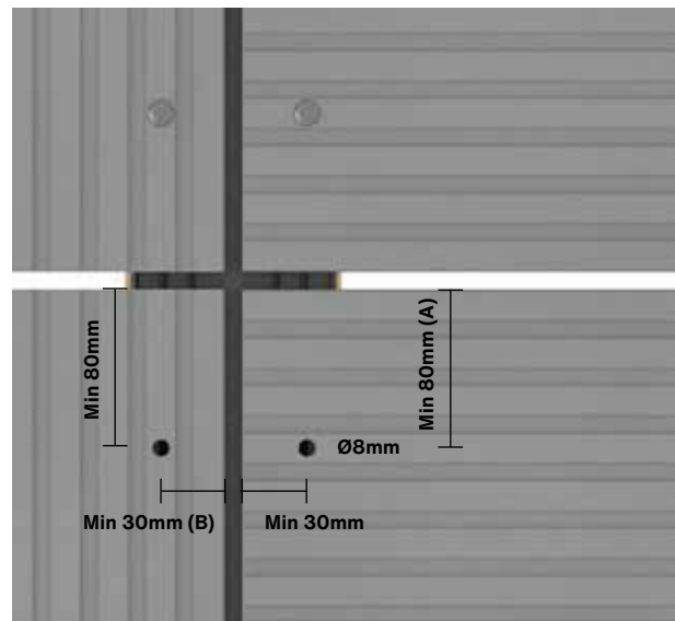
3 pav. Atstumai nuo „Swisspearl Patina Inline“ plokštės kraštų. DĖMESIO! Minimalus atstumas ir (arba) sekančios linijos viršus.
