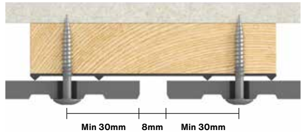
1 pav. Plokštės „Swisspearl Patina Inline“ tvirtinimas vertikaliaios siūlės vietoje.
