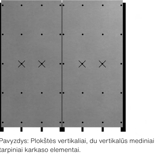
Paveikslėlis, kuriame nurodomas tinkamas varžtų montavimas. Fiksuoti tvirtinimo taškai pažymėti X.
