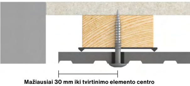
4 pav. Įjaustų „Swisspearl Patina Inline“ plokštės montavimas.
