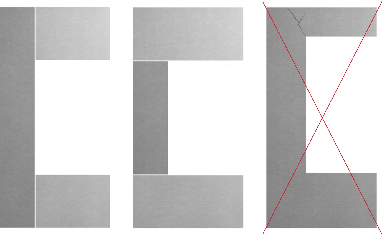
Teisingas „Swisspearl“ fasado plokščių montavimas ties langais, durimis ir kitomis angomis.
