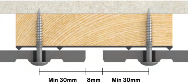
1 pav. Plokštės „Swisspearl Patina Inline“ tvirtinimas vertikalios siūlės vietoje.
