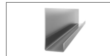
Swisspearl Plank Connect gala profils Krāsots alumīnijs Biezums 1,0 mm Garums 3000 mm
