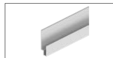
Swisspearl Plank Connect loga profils Profils, ekstrudēts alumīnijs Biezums 1,1 mm Garums 3000 mm
