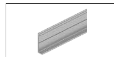
Swisspearl Plank Connect vertikālais sākuma profils Ekstrudēts alumīnijs Biezums 1,1 mm Garums 3000 mm
