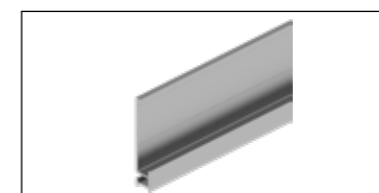
Swisspearl Plank Connect sākuma profils Ekstrudēts alumīnijs Biezums 1,1 mm Garums 3000 mm
