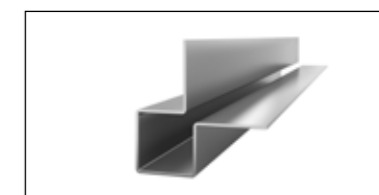
Swisspearl ārējā stūra profils Mazs, krāsots alumīnijs Biezums 1,0 mm Garums 3000 mm
