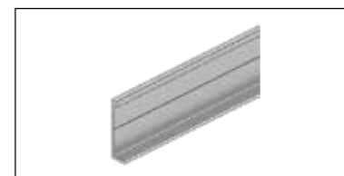
Swisspearl Plank Connect vertikālais sākuma profils Ekstrudēts alumīnijs Biezums 1,1 mm Garums 3000 mm
