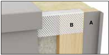
4. attēls A. Swisspearl Plank Connect nobeiguma profils B. Swisspearl ventilācijas profils
