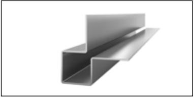
Swisspearl mazais ārējais stūris Krāsots alumīnijs Biezums 1,0 mm Garums 3000 mm
