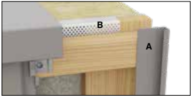
7. attēls. A. Swisspearl Plank Connect nobeiguma profils B. Swisspearl ventilējams profils
