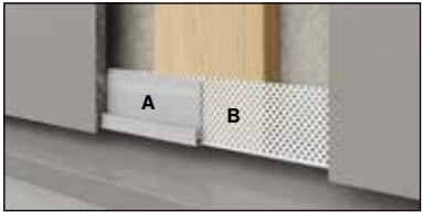
7. attēls. A. Swisspearl Plank Connect sākuma profils B. Swisspearl ventilācijas profils
