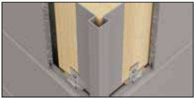
1. attēls Swisspearl ārējā stūra mazais profils
