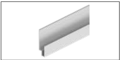
Swisspearl Plank Connect loga profils Profils, ekstrudēts alumīnijs Biezums 1,1 mm Garums 3000 mm
