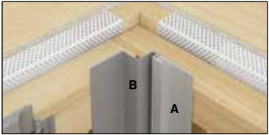
3. attēls A. Swisspearl Plank Connect sākuma profils B. Swisspearl iekšējais stūris
