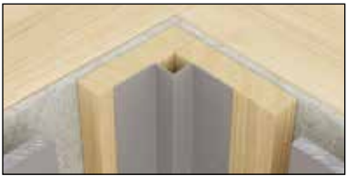
3. attēls Swisspearl iekšējā stūra profils
