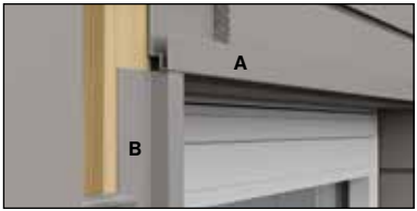
5. attēls A. Swisspearl Plank Connect loga profils B. Swisspearl ārējā stūra mazais profils
