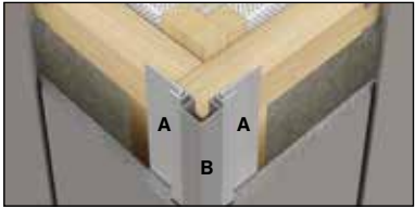
1. attēls A. Swisspearl Plank Connect sākuma profils B. Swisspearl mazais ārējais stūris
