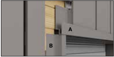
4. attēls A. Swisspearl Plank Connect loga profils B. Swisspearl ārējā stūra profils
