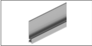
„Swisspearl Plank Connect“ pradžio profilis Ekstruduotas aliuminis Storis 1,1 mm Ilgis 3000 mm
