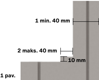
„Swisspearl Plank Connect“ lango aptaisymo sprendimas
