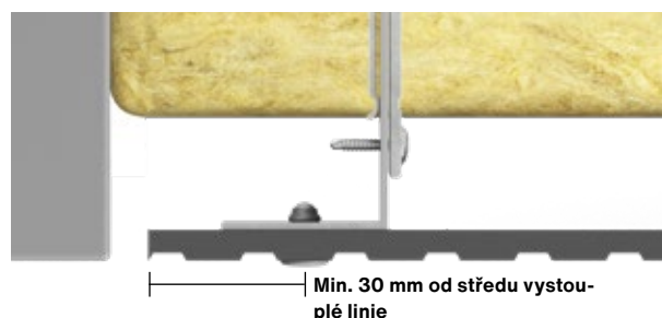
Obr. 4 Instalace přiřezávaných desek Swisspearl Patina Inline.
