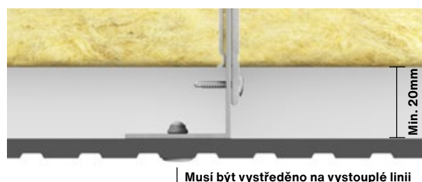
Obr. 2 Instalace panelů Swisspearl Patina Inline na L-profil.
