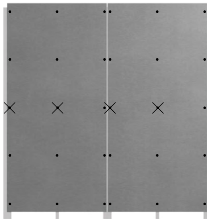
Příklad: svisle montované desky s jedním hliníkovým meziprofitem
