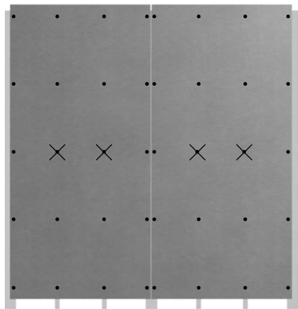
Příklad: svisle montované desky se dvěma hliníkovými meziprofily
