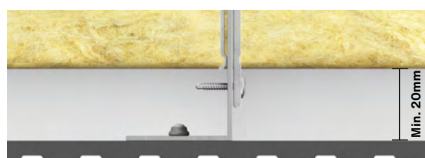
Obr. 2 Instalace panelů Swisspearl Patina Inline na L-profil.
