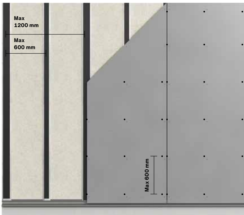
Fasádní desky Swisspearl instalované na svislých profilech VFL
