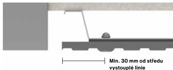
Obr. 4. Instalace přiřezávaných desek Swisspearl Patina Inline.
