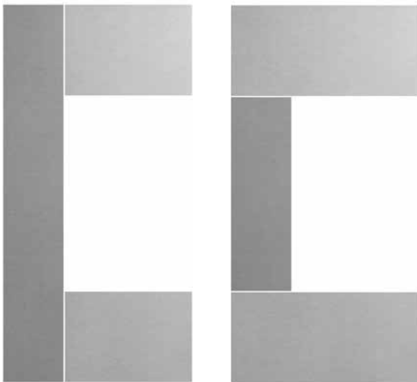
Obr. 2. Správná instalace fasádních desek Swisspearl kolem oken, dveří a stavebních otvorů.
