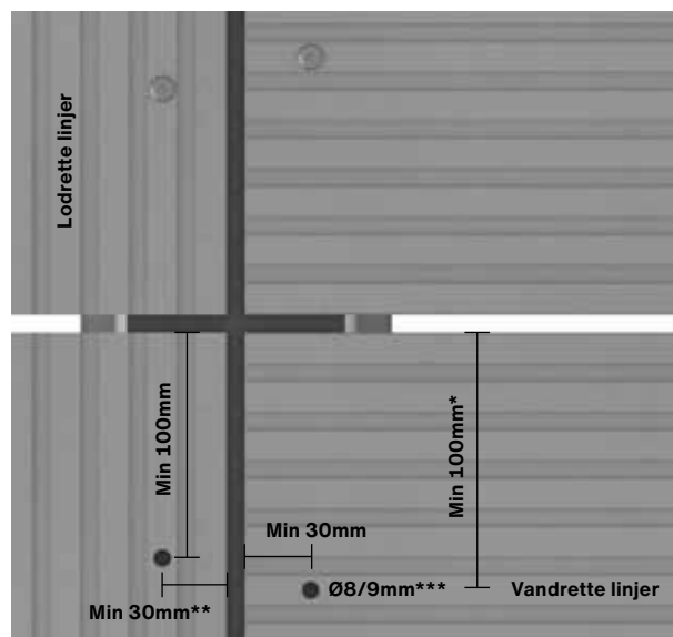
Obr. 3. Vzdálenosti od hran u desek Swisspearl Patina Inline. Upozornění! Min. vzdálenost a/nebo nejbližší následující horní linie. ***9mm vrták pro nýty a 8mm vrták pro vruty.
