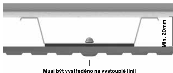
Obr. 2. Instalace panelů Swisspearl Patina Inline na středový profil.
