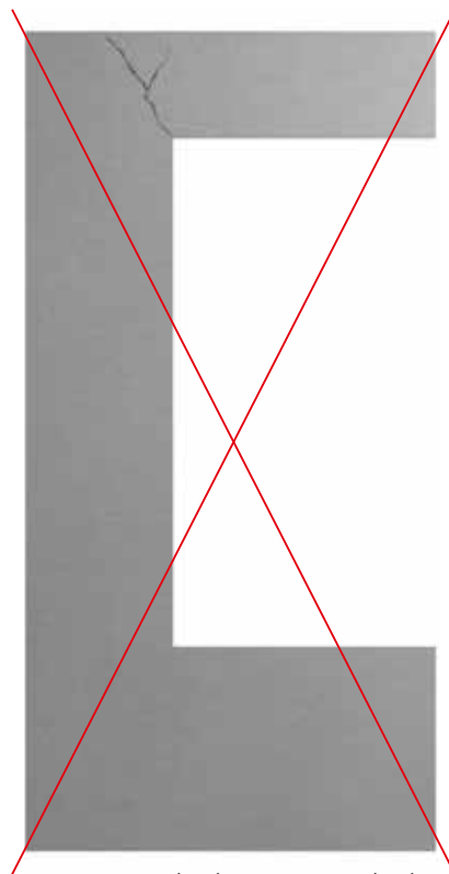
Obr. 3. Nesprávná instalace fasádních desek Swisspearl kolem oken, dveří a stavebních otvorů.
