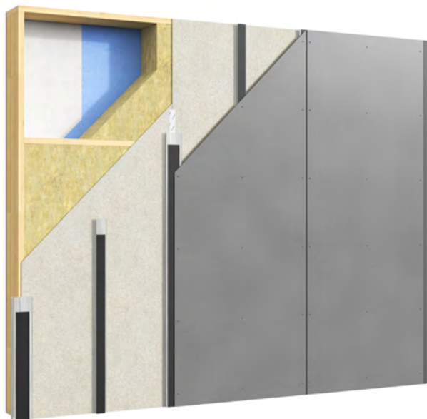
Lehká stěna se svislými ocelovými profily VFL
