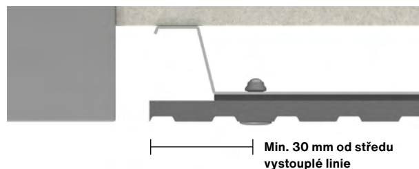
Obr. 4. Instalace přirézávaných desek Swisspearl Patina Inline.
