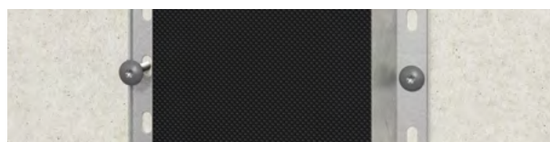
Obr. 2 Kluzné body: Profily Swisspearl VFL se montují upevňovacími prvky vkládanými doprostřed oválných otvorů.
