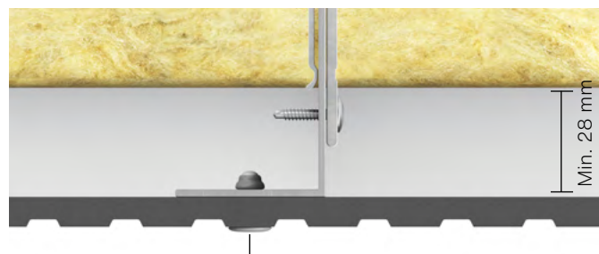
Fig. 2. Doit être centré sur la ligne supérieure Pose de panneaux Swisspearl Patina Inline sur profilé en L.
