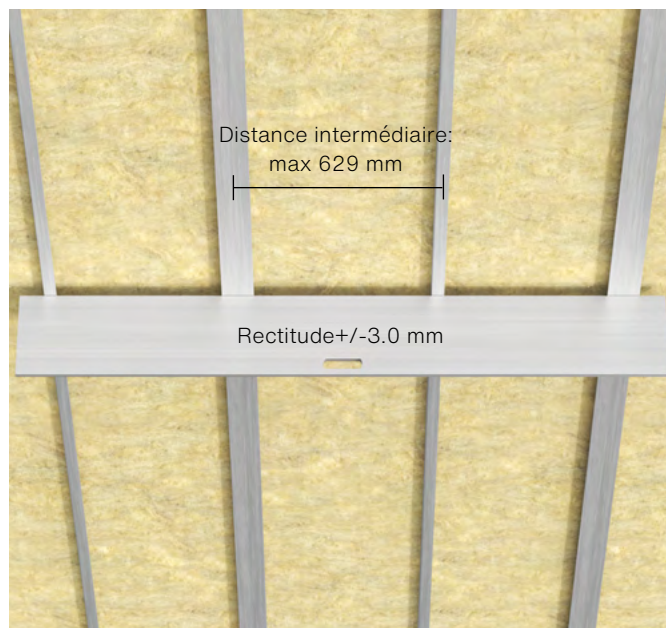
Rectitude de la construction sous-jacente
