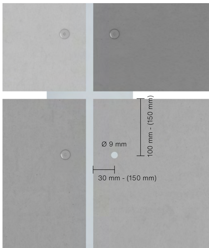
Exemple d'une construction sous-jacente verticale
