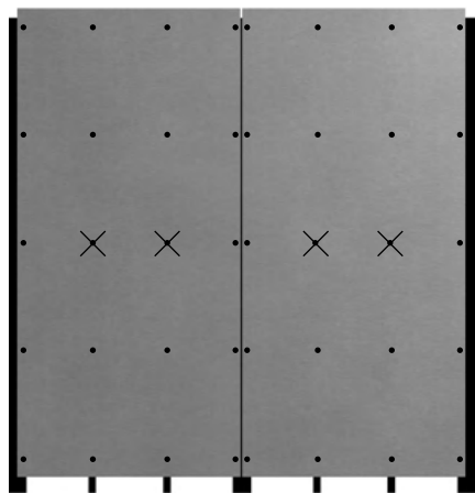
Exemples: Panneaux montés verticalement avec deux lattes intermédiaires en bois
