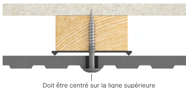
Fig. 2. Pose des panneaux Swisspearl Patina Inline NXT sur latte intermédiaire.
