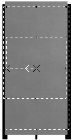
Illustration de la pose correcte des vis. Les points fixes sont marqués d'un x.
