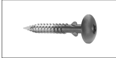
Vis de façade à ailettes pour support bois Swisspearl SCR-WW 4,9 x 38 mm Acier inoxydable A2 (Gamme Swisspearl Patina NXT)
