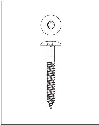
Fassadenschraube, Flachrundkopf Ø12 mm, T20 4,8x38 / K12 mm.
