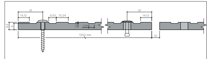
Patina Inline NXT | Befestigung immer mittig am Rillenberg!
