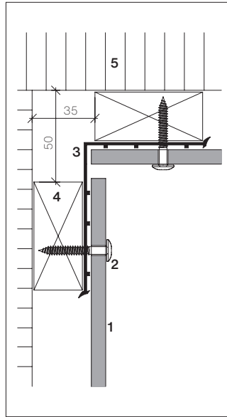
Innenecken
