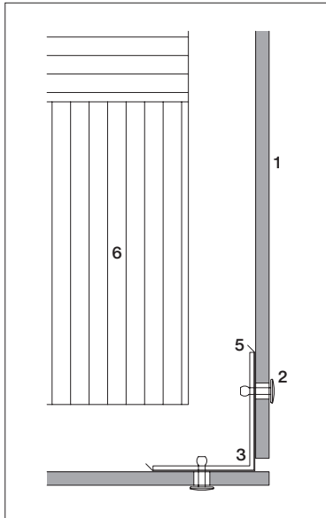
Außenecken
