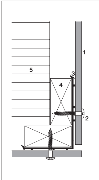
Außenecken
