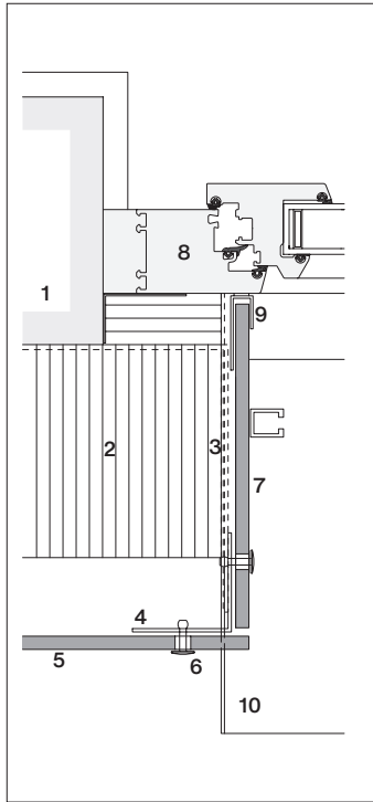
Fensteranschluss
