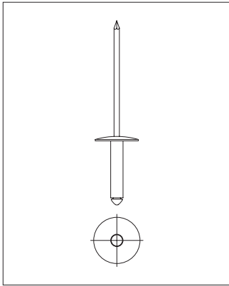
Fassadenniete, Nietkopf \varnothing 15 mm 4x18-K15
