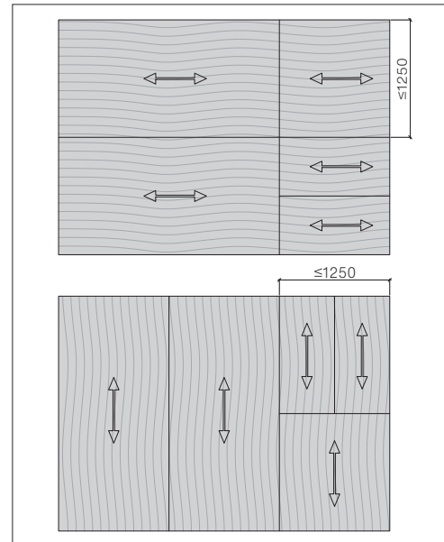
Fassadenansicht – Farbseite
