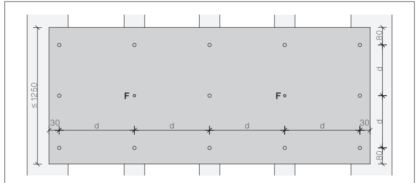
Patina NXT liegend
