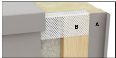
Foto 4 A. Swisspearl Plank Connect Eindprofiel B. Swisspearl Ventilatieprofiel
