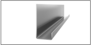
Swisspearl Plank Connect Eindprofiel Gepoedercoat aluminium Dikte 1.0 mm Lengte 3000 mm
