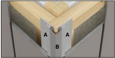
Foto 1 A. Swisspearl Plank Connect Startprofiel B. Swisspearl Buitenhoek Klein
