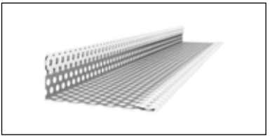
Swisspearl Ventilatieprofiel Brut aluminium Dikte 0.6 mm Lengte 3000 mm
