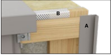
Foto 7 A. Swisspearl Plank Connect Eindprofiel B. Swisspearl Ventilatieprofiel
