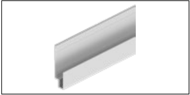
Swisspearl Plank Connect Raamprofiel Geëxtrudeerd aluminium Dikte 1,1 mm Lengte 3000 mm
