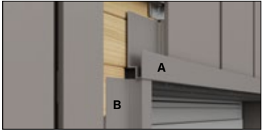
Foto 4 A. Swisspearl Plank Connect Raamprofiel B. Swisspearl Buitenhoekprofiel
