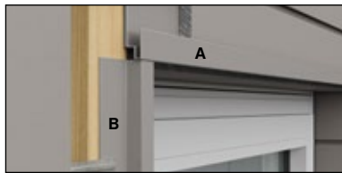
Foto 5 A. Swisspearl Plank Connect Raamprofiel B. Swisspearl Buitenhoekprofiel Klein
