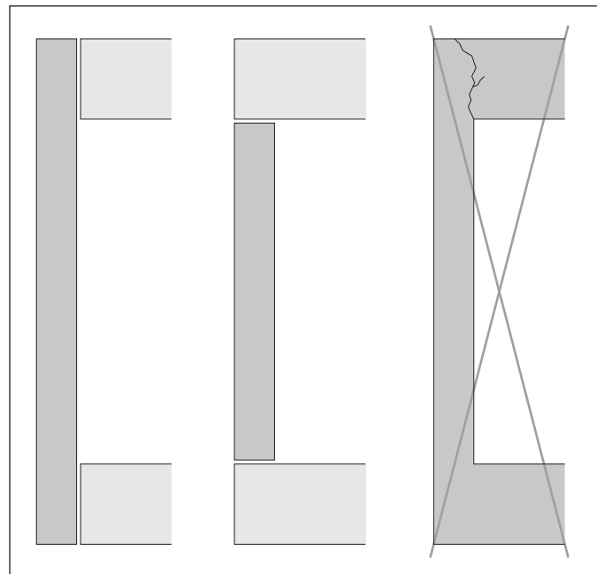
Richtige Anordnung von Patina NXT-Fassadenplatten bei Fenstern, Türen und anderen Öffnungen
