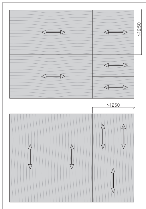
Ansicht fassadenseitig (Farbseite)
