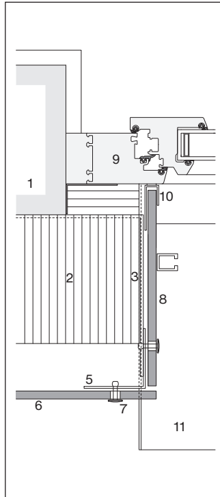
Patin NXT-Leibungsplatte 8mm
