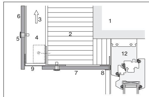
Fenstersturz mit Patina NXT-Untersichtplatte
