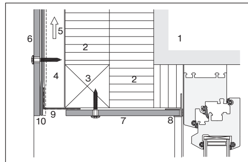
Fenstersturz mit Partin NXT-Untersichtplatte
