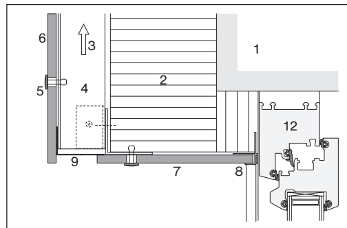
Fenstersturz mit Patina NXT-Untersichtplatte
