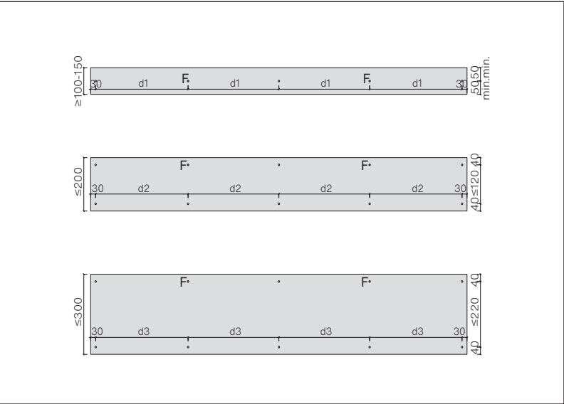
Festpunktanordnung bei einer horizontalen Patina NXT-Streifenverlegung. Bei einer Plattenhöhe von \leq 300 mm darf der vertikale Randabstand auf min. 40 mm verringert werden.
