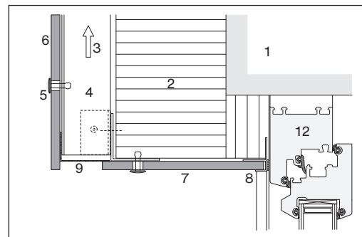
Linéau de fenêtre avec plaque Patina NXT
