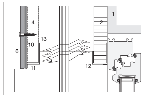
Linéau de fenêtre avec stores
