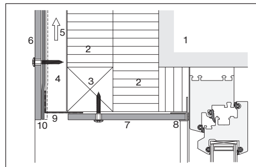
Linéau de fenêtre avec plaque de sous-face Patina NXT
