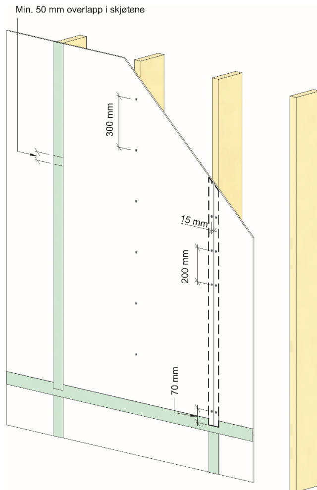
Fig. 1 Swisspearl Windstopper montert på yttervegg med trestendere med tape over alle plateskjøtene.
