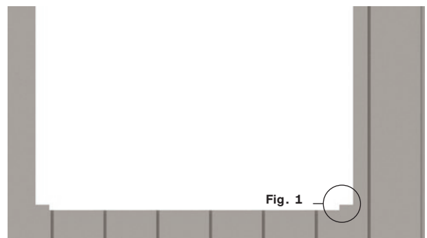
Swisspearl Plank Connect vindusløsning
