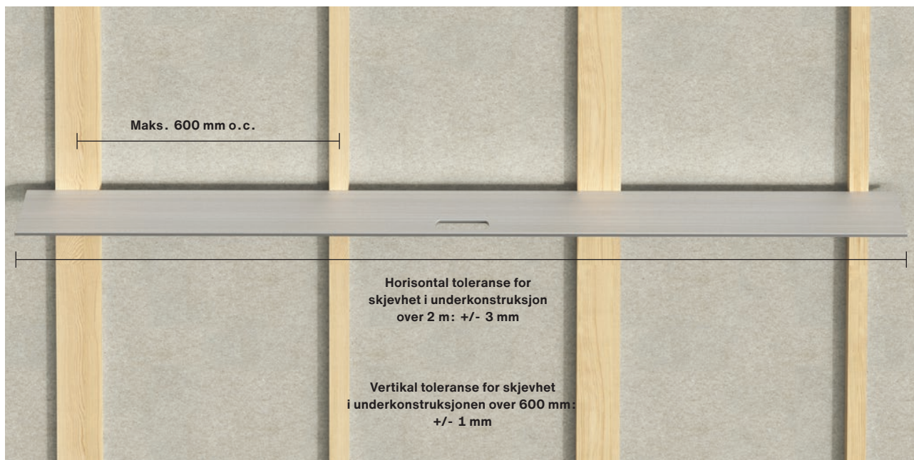
Skjevhet i underkonstruksjon
