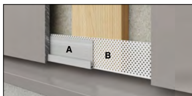
Foto 7 A. Swisspearl Plank Connect Startprofiel B. Swisspearl Ventilatieprofiel
