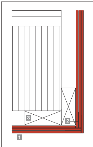
vaakaleikkaus, kulmapeltiritkaisu
