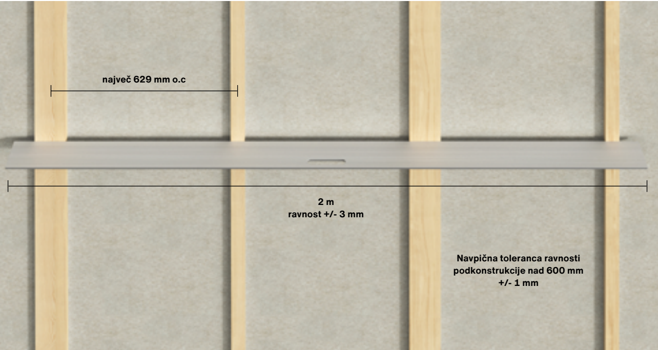
Ravnost podkostrukcije
