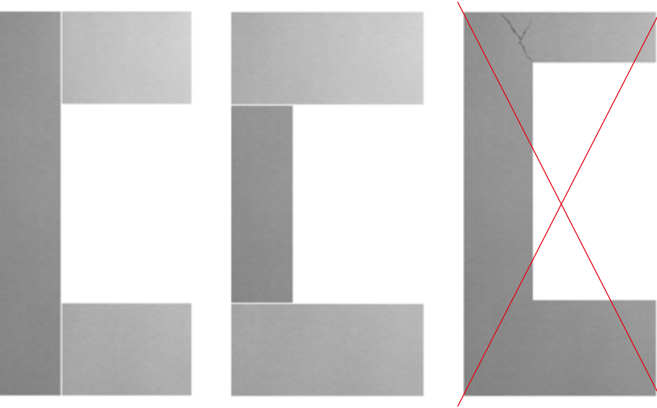
Pravilna namestitev fasadnih plošč Swisspearl pri oknih, vratih in odprtinah.
