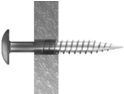
X : Premer pritrdilne luknje Ø 5 do 5,5 mm.
