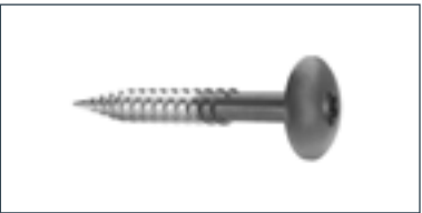
Fasadni vijak Swisspearl za les SCR-W 4,8 x 30/38/44 mm Nerjavno jeklo A2 (Linija Swisspearl Patina)
