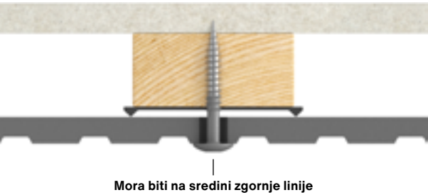
Slika 2: Namestitev Swisspearl Patina Inline na vmesno letev.
