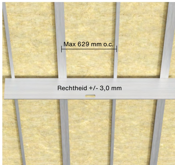
Rechtheid van de achterconstructie
