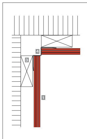
Kreuzprofil, Steghöhe 18 mm
