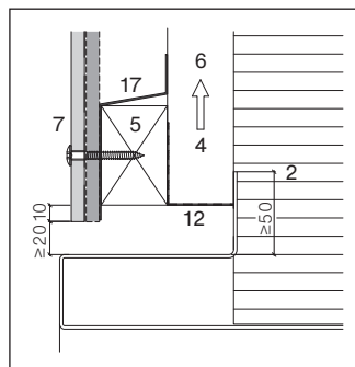
Linéau avec huisserie
