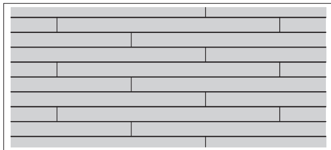
Jointes verticales décalés \frac{1}{3}
