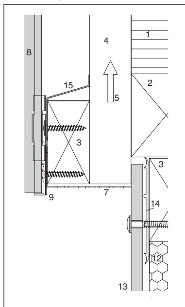
Ossature bois/bois
