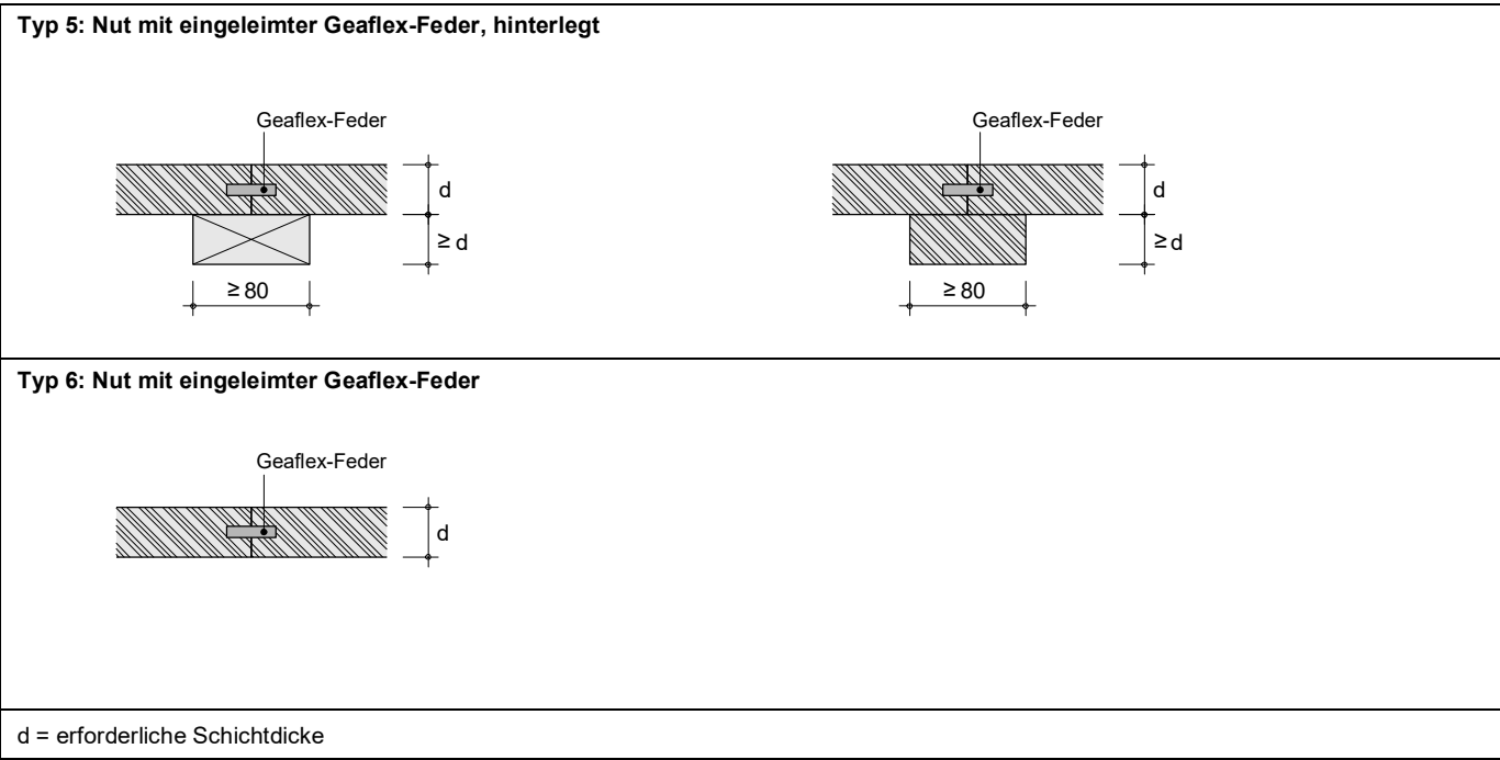
Abbildung 5b: Fugentypen für Duripanel, Cemspan und Cemcolor (Einsatz gemäss Abb. 4)
